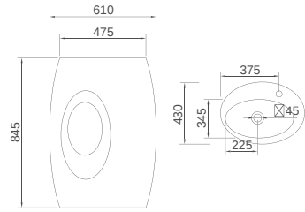
R-1388 Size: 610x430x845mm
