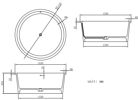
B064-A Size: 1520x1520x610mm
