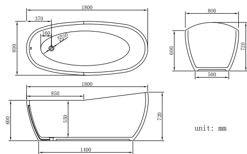
B063-A Size: 1800x800x720mm
