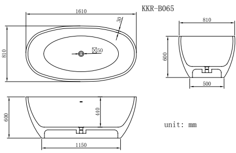
B065 Size: 1610x810x600mm
